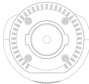
仰视图
