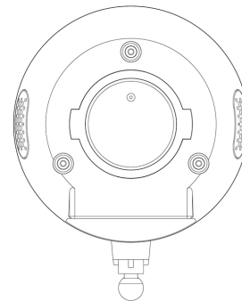
仰视图
